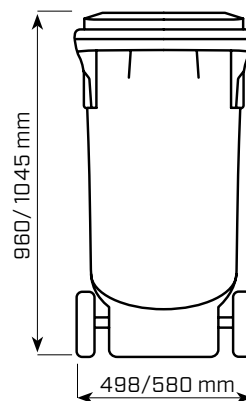
Rozměry nádoby 120/200 l
